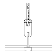
Perfil fineline T-15 Fineline form T-15
